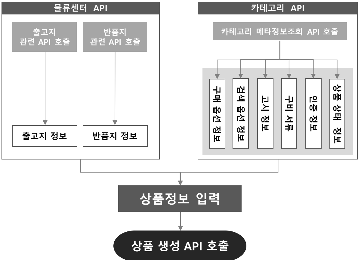
<[그림] 상품 생성 API 호출의 대략적인 흐름>
